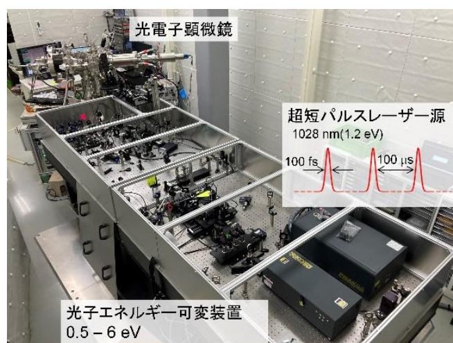
図2 フェムト秒幅のパルスレーザーを光源とする光電子顕微鏡（フェムト秒光電子顕微鏡）の外観写真（1 フェムト秒は 1000 兆分の 1 秒）。短い時間幅のレーザーパルスを利用することで、光のエネルギーを近赤外光から紫外光領域（0.5～6 eV）まで自在に変化させることができる。
