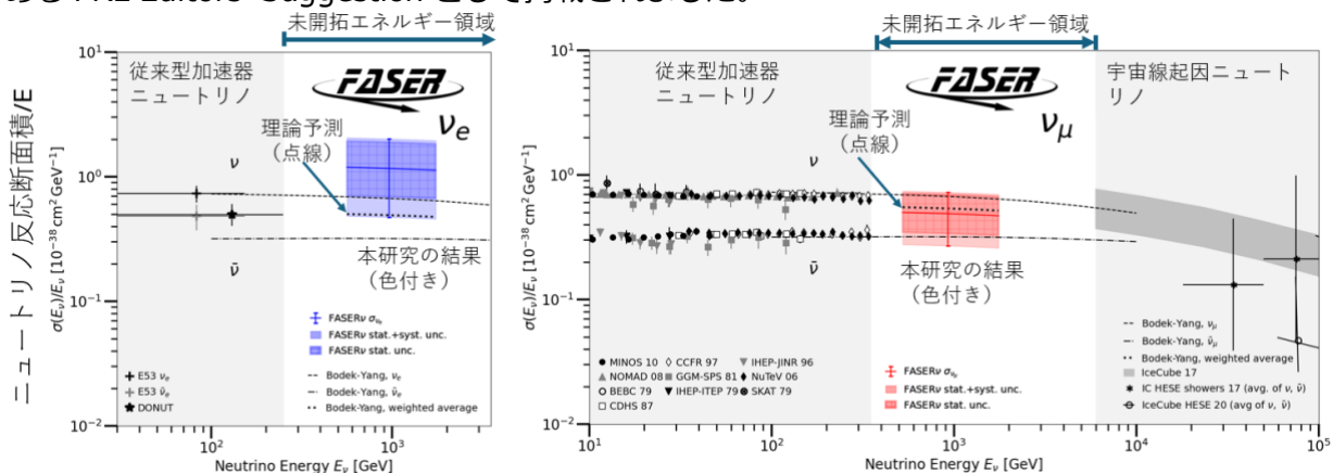
図1 電子ニュートリノ(青)とミューニュートリノ(赤)反応断面積測定結果
