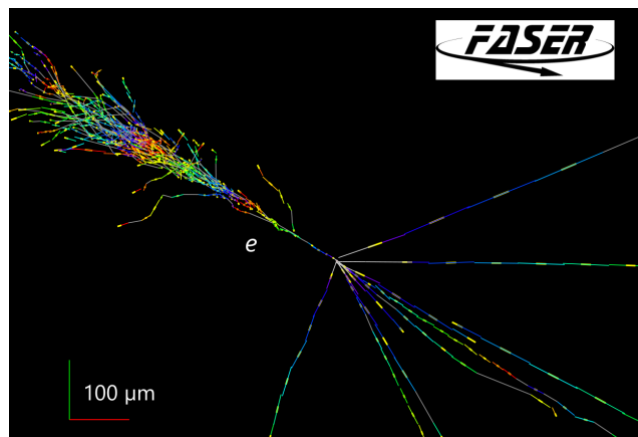
図 4 FASER v 検出器中で捕えた電子ニュートリノ反応事象のイベントディスプレイ。ニュートリノの進行方向から見たもので、左上に 1.5 TeV の電子と右下にその他の粒子が放出されていることが分かる。
