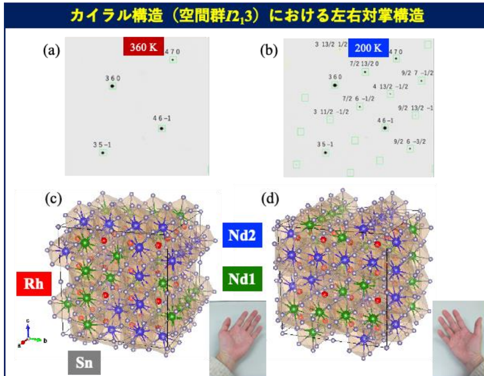
図 1 : (a) 360 K (87°C) と (b) 200 K (マイナス 73°C) で測定した放射光 X 線データ。低温で新しい回折ピークが現れ、結晶構造が変化したことがわかる。(c)(d) この放射光 X 線回折実験によって決定した結晶構造 (VESTA による描画)。(c) を左手に対応させると、(d) は右手に相当する対掌のカイラル対称結晶構造になっている。ネオジウムは 2 種類 (緑色の Nd1 と青色の Nd2) 存在し、それらが一次的に並んでいる鎖が左回り、あるいは右回りで配置するように見える。左右それぞれの結晶構造は空間反転対称性が破れている。
