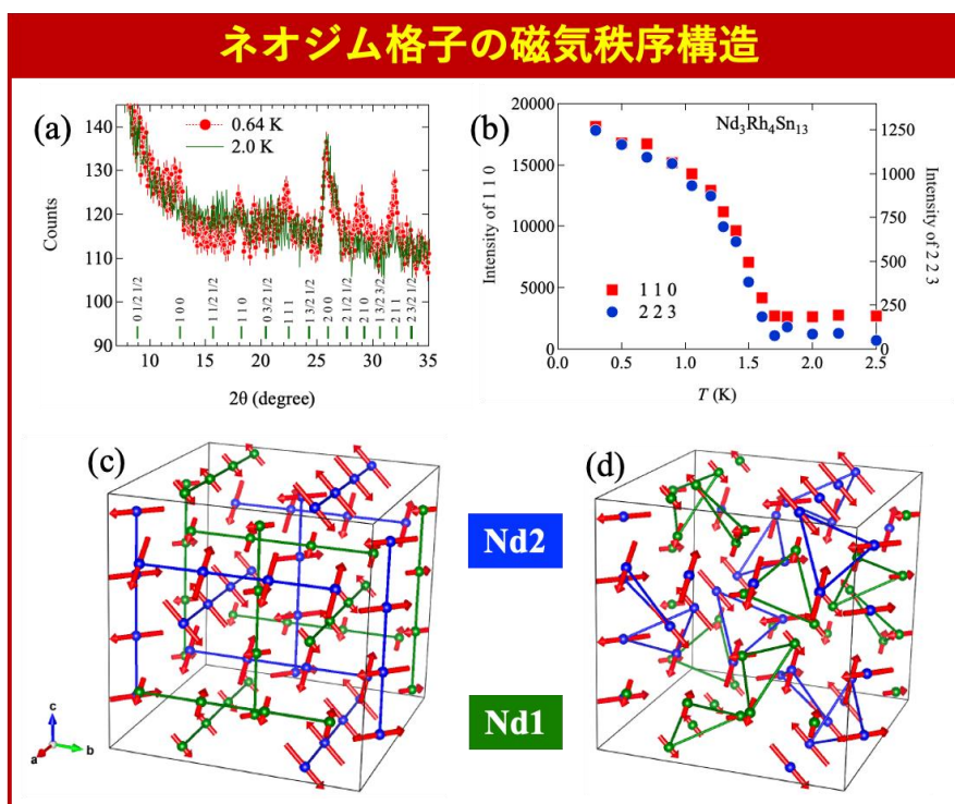
図 2 : (a) 0.64 K (約マイナス 272°C) と 2 K (マイナス 271°C) での中性子回折パターンを示す。(b) 中性子回折強度の温度依存性。1.65 K 以下で反強磁気秩序構造が生じていることを示している。(c) 中性子回折から導いた反強磁気秩序構造。ネオジムの一次元鎖で磁気モーメントは交替配列している。(d) 見方を変えると 1 次元鎖は三角格子で連結しており、磁気フラストレーション系の特徴を持っている。
