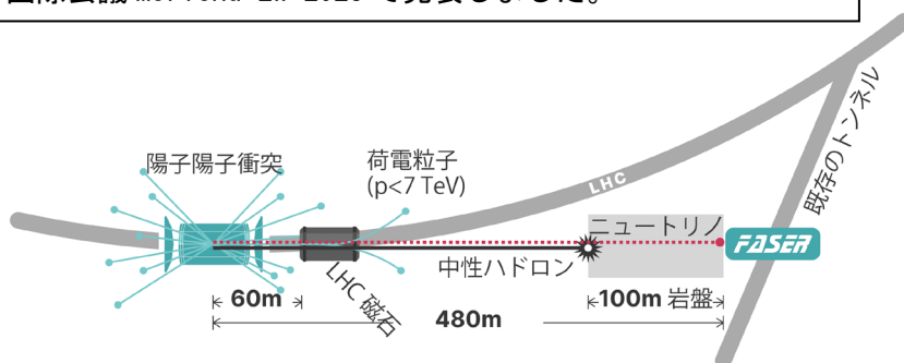
(右図) LHC の陽子衝突で生成したニュートリノをビーム軸方向 480m 地点に設置した FASER 検出器によって捕える様子。
