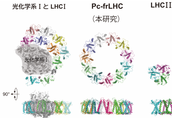
図 4：緑藻における光合成光捕集アンテナタンパク質の構造の比較
