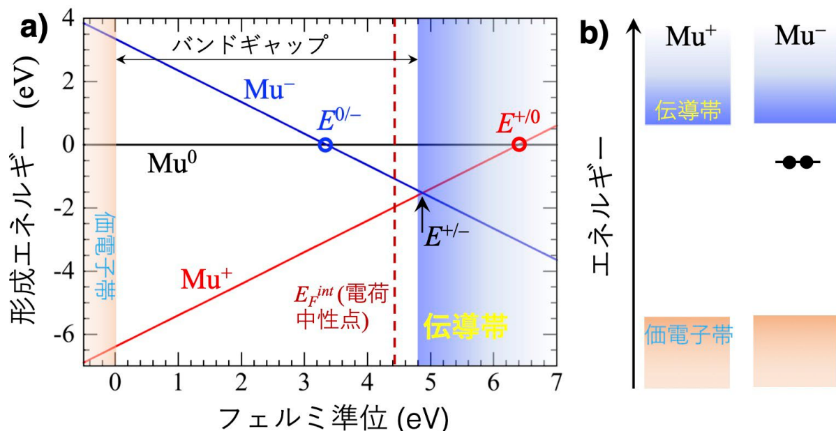
図 2 (a) \beta\text{-Ga}_2\text{O}_3 でのミュオン ( \text{Mu}^q , q=0,\pm 1 ) の形成エネルギー (注6) とフェルミエネルギーの関係図。 \text{H}^+ の形成エネルギーと \text{H}^0 の形成エネルギーの交点をドナー準位 ( E^{+/0} )、 \text{H}^- の形成エネルギーと \text{H}^0 の形成エネルギーの交点をアクセプター準位 ( E^{0/-} ) とし、最近提案された両極性モデル (注4) では、H (あるいは Mu) はこれらに対応した 2 つの準安定状態を同時に取り得ると仮定する。今回の実験結果はこのモデルとよく一致している。 E^{0/-} が伝導帯中に存在するため、対応する H (あるいは Mu) は常にイオン化 ( \text{H} \rightarrow \text{H}^+ + e^- ) して電子を供給する、つまり意図しない n 型伝導を引き起こす原因となることを意味する。また、 E^{0/-} が伝導帯に近い位置にある一方で、電荷中性点 E_F^{\text{int}} よりも低エネルギー側 (図で左側) にあることから、 E^{0/-} に対応する状態が実際にアクセプターとして機能し、伝導帯と電子のやりとりが可能であることを示唆している。 (b) ドナー ( \text{Mu}^+ = \text{Mu}_1 ) とアクセプター ( \text{Mu}^- = \text{Mu}_2 ) 準位に対応したバンド構造の模式図。 \text{Mu}^- は伝導帯と電子をやりとりし、一時的な \text{Mu}^0 状態を経由しながら高速で拡散する。
