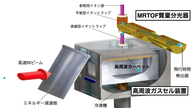
図 3 実験装置の概念図
