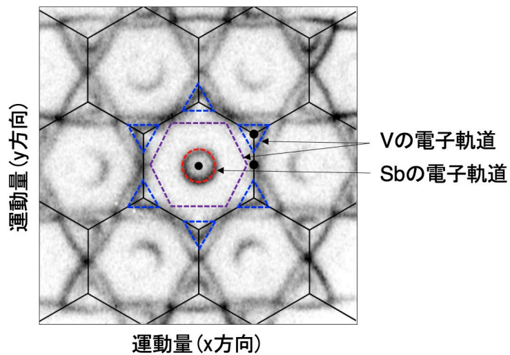
図4 \text{CsV}_3\text{Sb}_5 で測定した光電子強度。V(青や紫のガイドライン)や Sb(赤のガイドライン)に由来する電子構造を分離して観測することができます。
