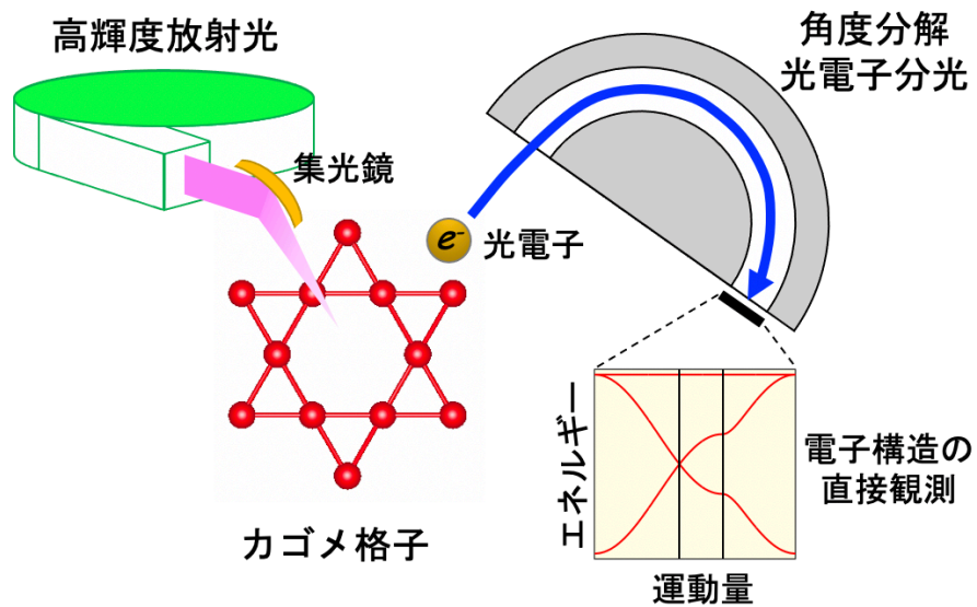
図2 カゴメ格子物質のマイクロ ARPES 測定概念図。ミクロン単位まで微小集光した高輝度放射光で試料上を走査し、局所電子構造を高運動量分解能で決定できます。
