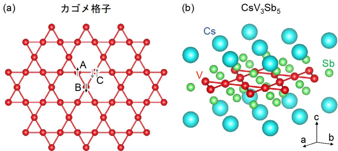
図1 (a)カゴメ格子と(b) \text{CsV}_3\text{Sb}_5 の構造の模式図。(a)中の矢印は、位置 A、B、C における電子スピンの向きを表しており、C では上向きと下向きのどちらにも定まらない、不安定な状態となります(注2参照)。
