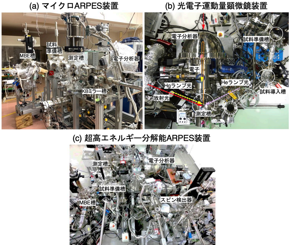
図3 (a) 高エネルギー加速器研究機構 フォトンファクトリーの BL-28 に建設されたマイクロ ARPES 装置、(b) 分子科学研究所 UVSOR の BL6U に建設された光電子運動量顕微鏡装置、(c) 東北大学に建設された超高分解能 ARPES 装置。
