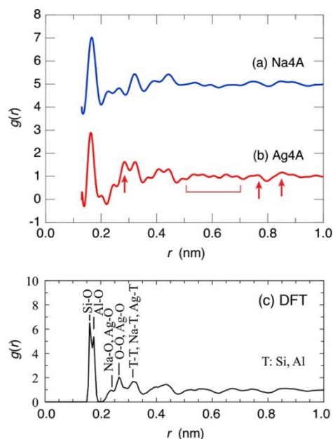
図3: HEXRD で求めた(a)銀を含まない、および(b)含む 4A 型ゼオライトの g(r) および (c) DFT 計算によって得られた結果
