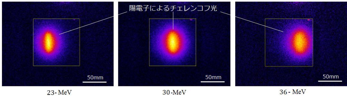
図 2. 正のミュオンビームを水に照射しながら高感度 CCD カメラを用いて撮像したミュオン崩壊陽電子のチェレンコフ光画像のミュオンビームエネルギーによる違い
