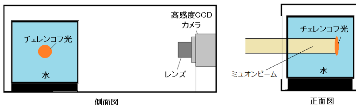
図 1. ミュオンビームイメージング法の概略図：側面図（左）と正面図（右）
