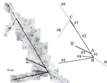
右図：伊吹イベントの写真乾板中の粒子の飛跡の写真。グザイマイナス粒子が窒素14原子核に吸収され、グザイ超原子核の形成した後に、ベリリウム10ラムダ核とベリリウム5ラムダ核へ崩壊しました。
