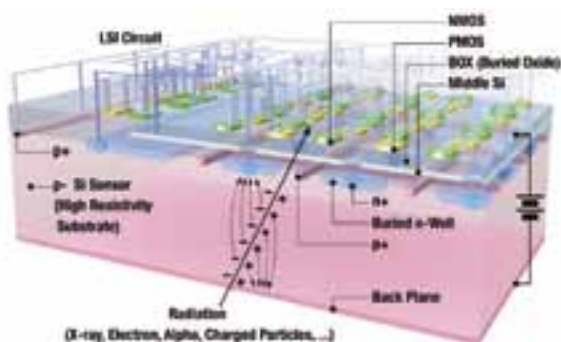
SOI 半導体で作る放射線センサー
