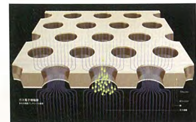
ガス電子増幅 (GEM) フィルム ©Rey.Hori
