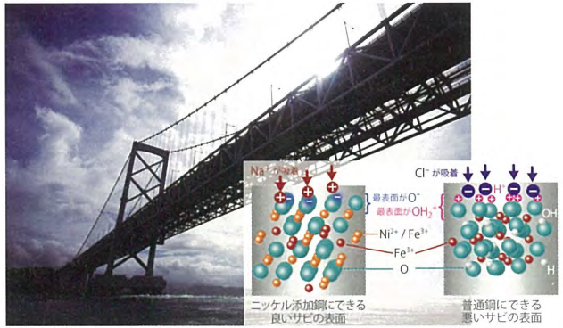
社会インフラ:長寿命な鋼材開発 耐食性を向上させる保護性サビの形成を発見、メカニズムを解明。鉄にニッケルを添加することで、内部まで侵入しない保護性サビが形成されることを放射光で解明した。
