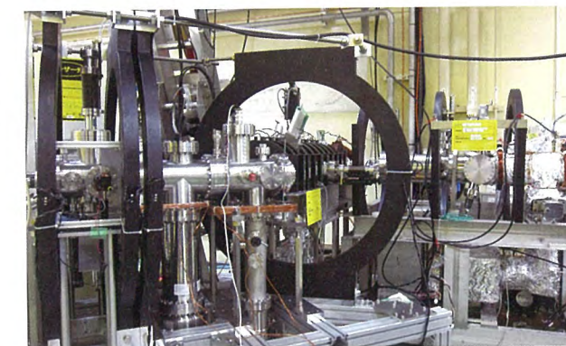
低速陽電子源
