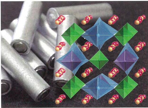
世界最高のリチウムイオン伝導率を示す超イオン伝導体 リチウムイオン電池の可燃性電解液に変わる固体電解質「超イオン伝導体」を発見。その結晶構造とイオン伝導経路を超高分解能粉末中性子回折装置を用いて解明した。
