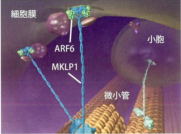
細胞内でタンパク質を輸送するしくみ フォトンファクトリーを利用して得られた微小管と細胞膜を橋渡すARF6(緑)とMKLP1(青)複合体の立体構造。
