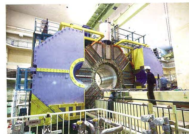
改造中の Belle II 測定器
