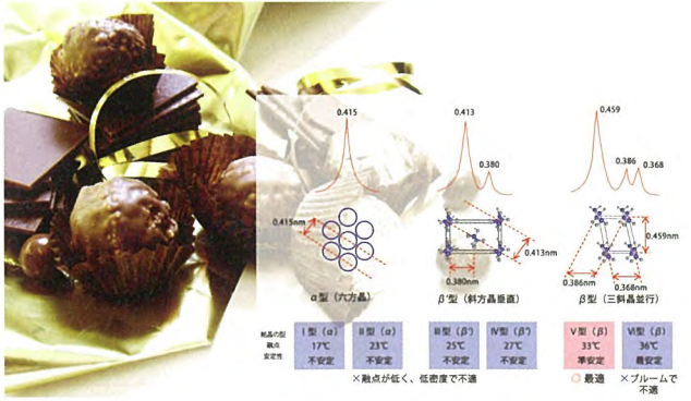
食品:食感の美味しさデザイン チョコレートの美味しさを決定するココアバター結晶多形変化を放射光回折実験で観測。これにより、美味しいチョコレートの品質を得るための条件を特定、製品造りに活かされている。
