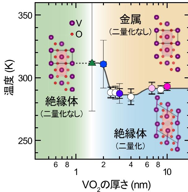
図 3: 今回の研究で決定した \text{VO}_2 ナノ構造の電子相図 1 nm 以下の極薄膜領域では、V イオンの二量化を伴わない絶縁体状態が現れています。
