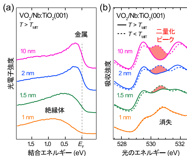
図 2: (a) 軟 X 線放射光を用いてその場で測定した VO 2 ナノ構造における光電子分光スペクトルの厚さ依存性
