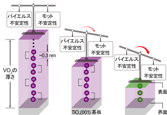
図 4: \text{VO}_2 ナノ構造に現れる新しい電子相の発現機構 \text{VO}_2 におけるモット不安定性とパイエルス不安定性の均衡がサイズ効果により崩れ、二量化を伴わないモット絶縁相が極薄膜領域に現れます。これは、強相関電子が 2 次的に閉じ込められることで強相関効果（モット不安定性）が強くなる一方で、V イオン二量体の形成効果（パイエルス不安定性）が弱くなるため、あるサイズ極限でモット不安定性が支配的になるためであると考えられます。
