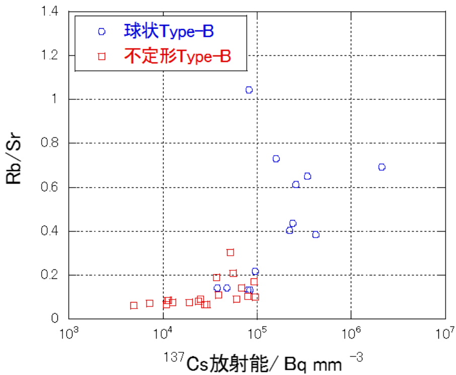
図4：マイクロビーム X 線を用いた蛍光 X 線分析により得られた \text{Rb/Sr} 比と ^{137}\text{Cs} 放射能の関係。
