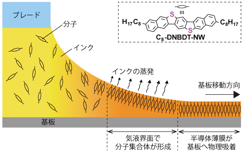
図1 印刷プロセスを用いた有機半導体単結晶薄膜の製造手法。基板の上に保持された半導体インクの表面では、多数の分子が自ら集合し、薄膜を形成する。インク表面で得られた薄膜は、インクの乾燥に伴い基板の上に物理吸着する。
