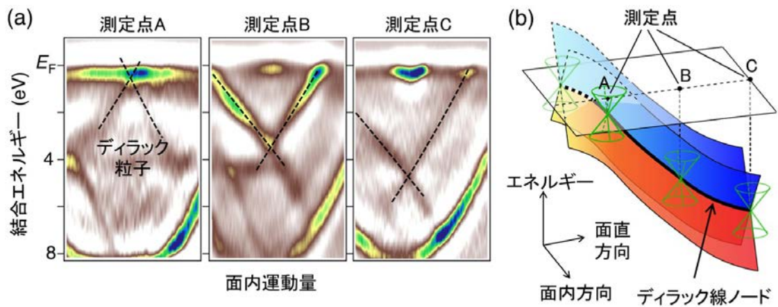
図 3: (a)角度分解光電子分光によって得られた、(b)に示した3ヶ所の測定点 (A, B, C)における AlB 2 のバンド分散。ディラック電子によるX字型の直線的なバンド分散が観測され、それがC→Aと移動すると、高いエネルギー側へシフトしていることがわかる。(b) AlB 2 における線ノード型のディラック粒子のエネルギー状態の模式図。
