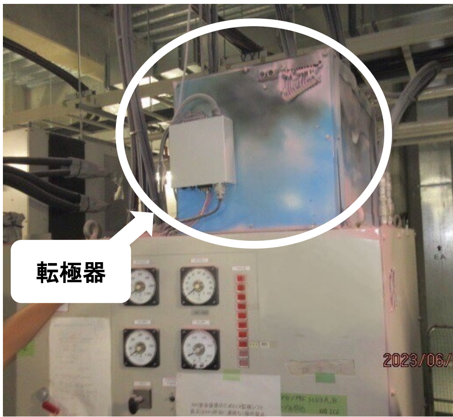
転極器正面
